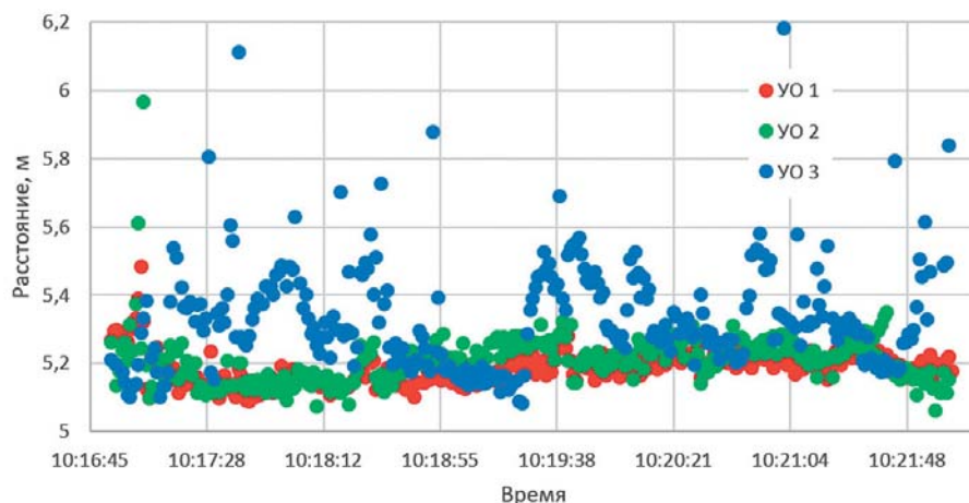
Рис. 2 Измерение расстояния при положении испытателя в одной точке с изменением положения устройства оповещения (для трех устройств)
