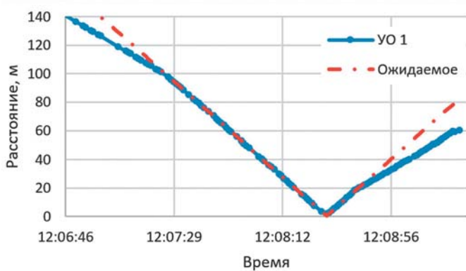
Рис. 4 Измерение расстояния при перемещении устройства оповещения с изменением скорости
