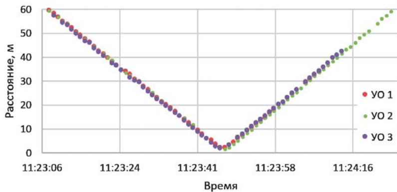
Рис. 3 Измерение расстояния при равномерном перемещении трех устройств оповещения через место установки базовой станции
